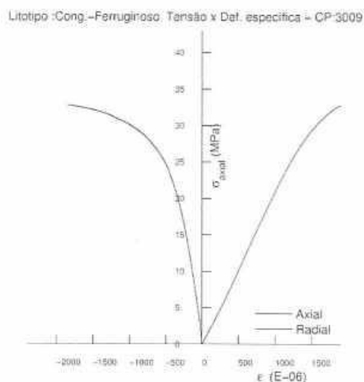
Figura 5.33 - Diagrama tensão axial versus deformação específica axial e radial do corpo de prova 3009.
