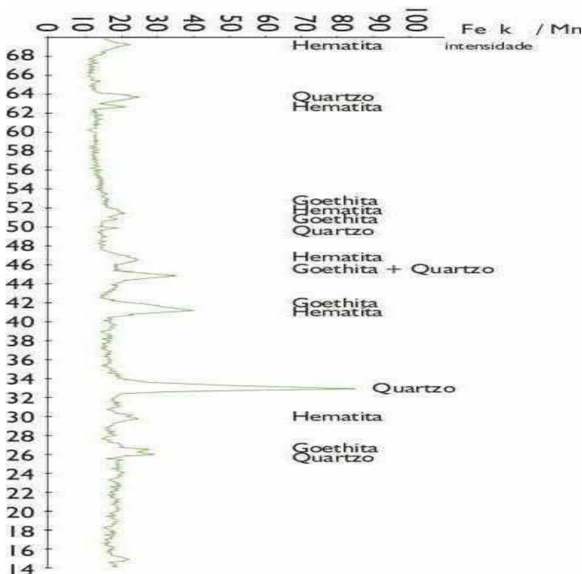
Figura 5.7 - Espectro da análise de difração de raios-X do conglomerado ferruginoso laterítico.
