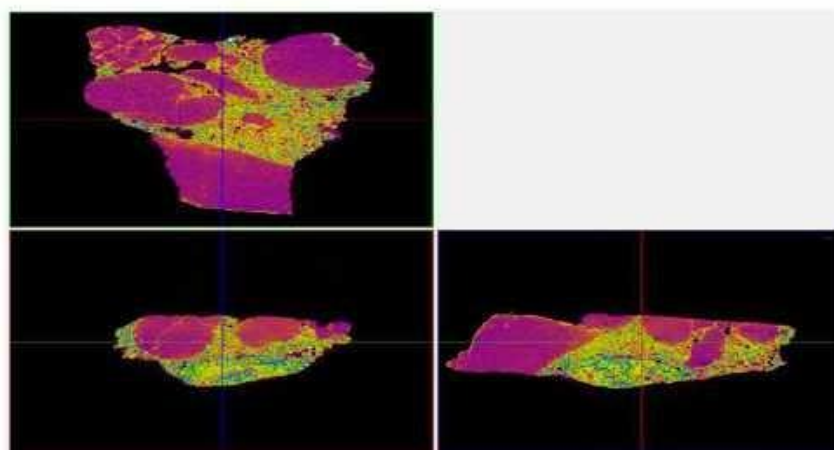
Figura 5.19 – Microtomografia computadorizada com raio X - vista bidimensional com distribuição dos poros.
