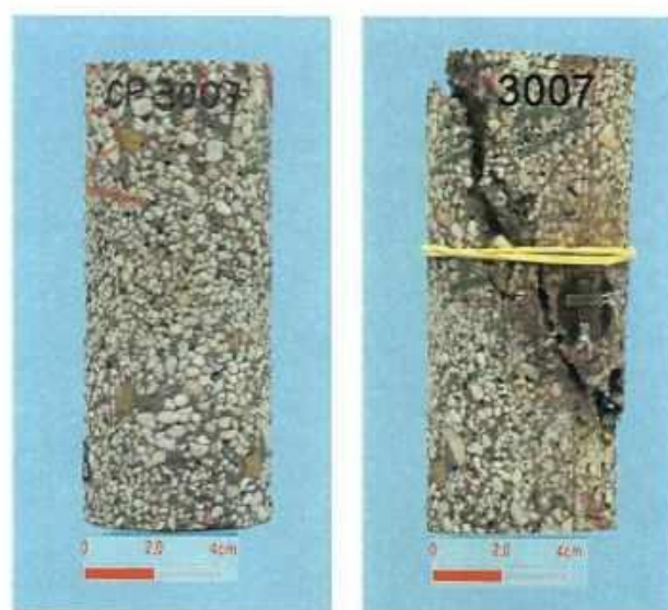
Figura 5.25 - CP 3007 antes e após o ensaio de compressão uniaxial.
