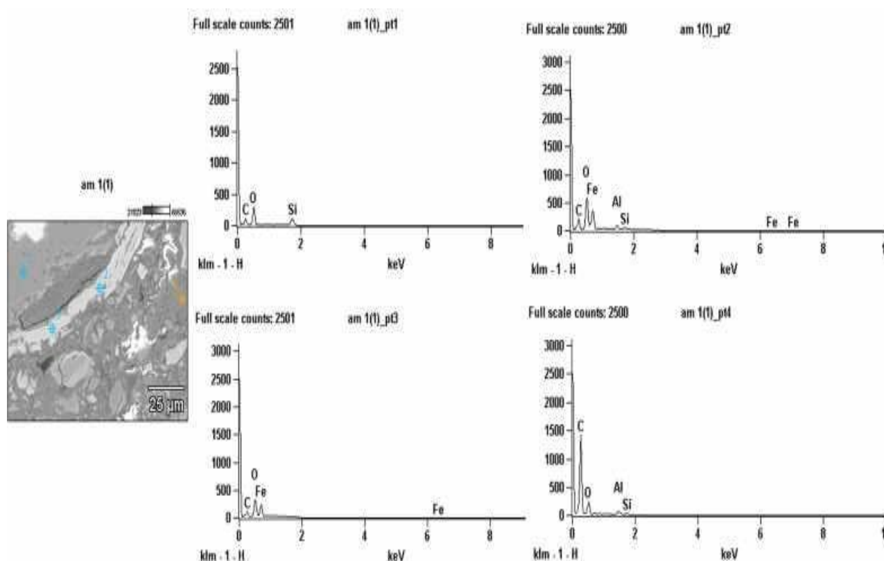
Figura 5.14 - Perfil pelos pontos 1,2,3 e 4 com os respectivos elementos químicos presentes: am 1 = C, O e Si = quartzo - am 2 = C, O, Fe, Al e Si = óxido de ferro + quartzo - am3 = C, O e Fe = óxido de ferro puro – am4 = C, O, Al e Si = óxido de alumínio.
