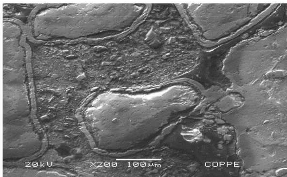
Figura 5.13 - Fotomicrografia MEV evidenciando em plano mais marcante os grãos de quartzo maiores envolvidos por uma fração/película de óxido ferruginoso. Entre um grão e outro, pode ser observado o cimento ferruginoso, no qual ocorrem disseminados finíssimos grãos de quartzo.
