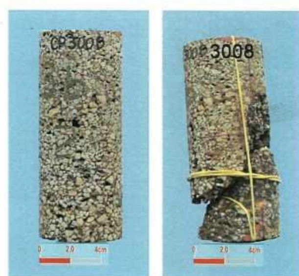
Figura 5.26 - CP 3008 antes e após o ensaio de compressão uniaxial.
