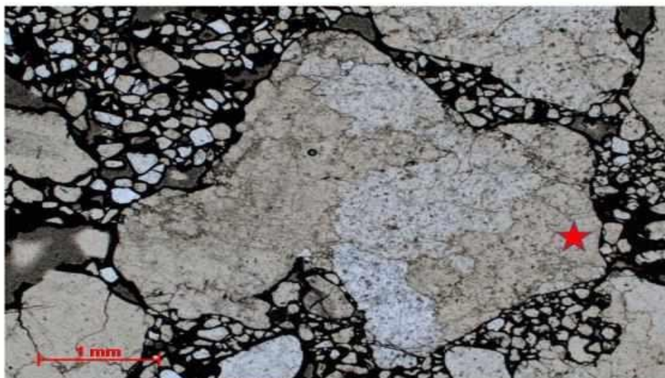
Figura 5.10 - Microfotografia com luz polarizada de detalhe do conglomerado ferruginoso laterítico, onde pode ser observado que o cimento engloba partículas muito finas de frações quartzosas, e assim estabelecendo uma maior área de contato entre diferentes materiais, no caso, cimento e grãos da matriz, gerando assim maior área de microdescontinuidades e consequente maior microporosidade, com reflexos nos índices físicos da rocha.
