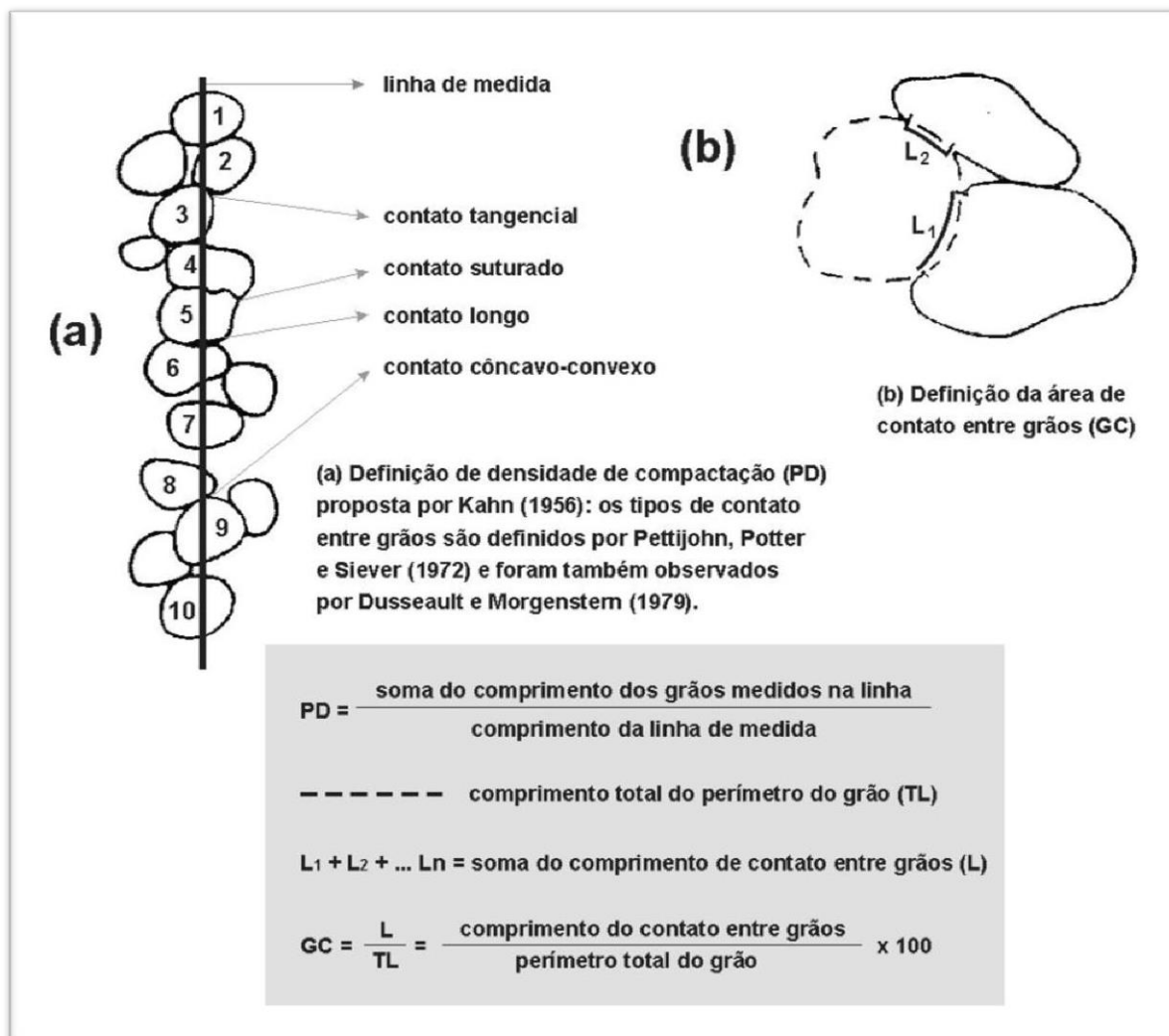
Figura 2.10 - Definição de densidade de compactação.
