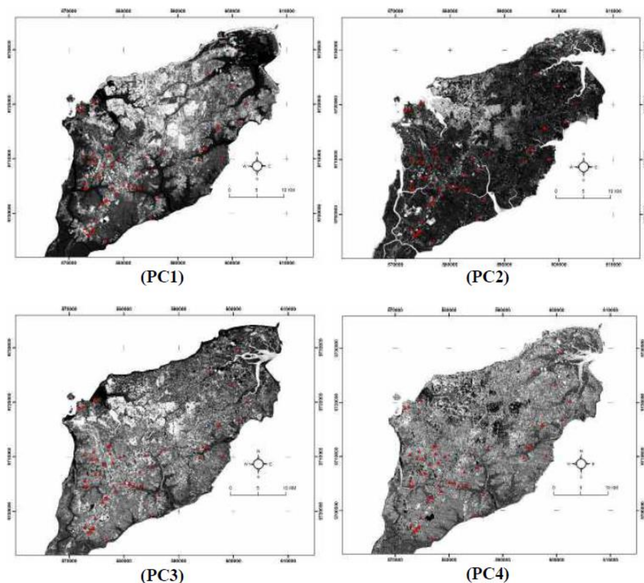
Figura 5.5 - Mosaico das principais componentes das cenas 220/62 e 221/62 geradas a partir dos canais originais TM 1-3-4-5. Minerais do grupo do óxido de ferro estão destacados como regiões claras na PC3 e como regiões escuras na PC4. Triângulos vermelhos correspondem às jazidas/pontos/lavras cadastradas.
