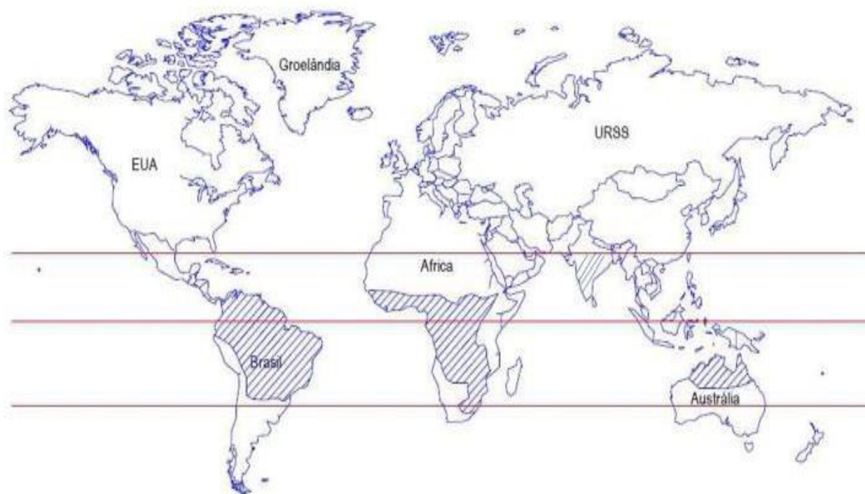
Figura 2.3 - Mapa mundial mostrando as regiões de ocorrência de solos lateríticos.
