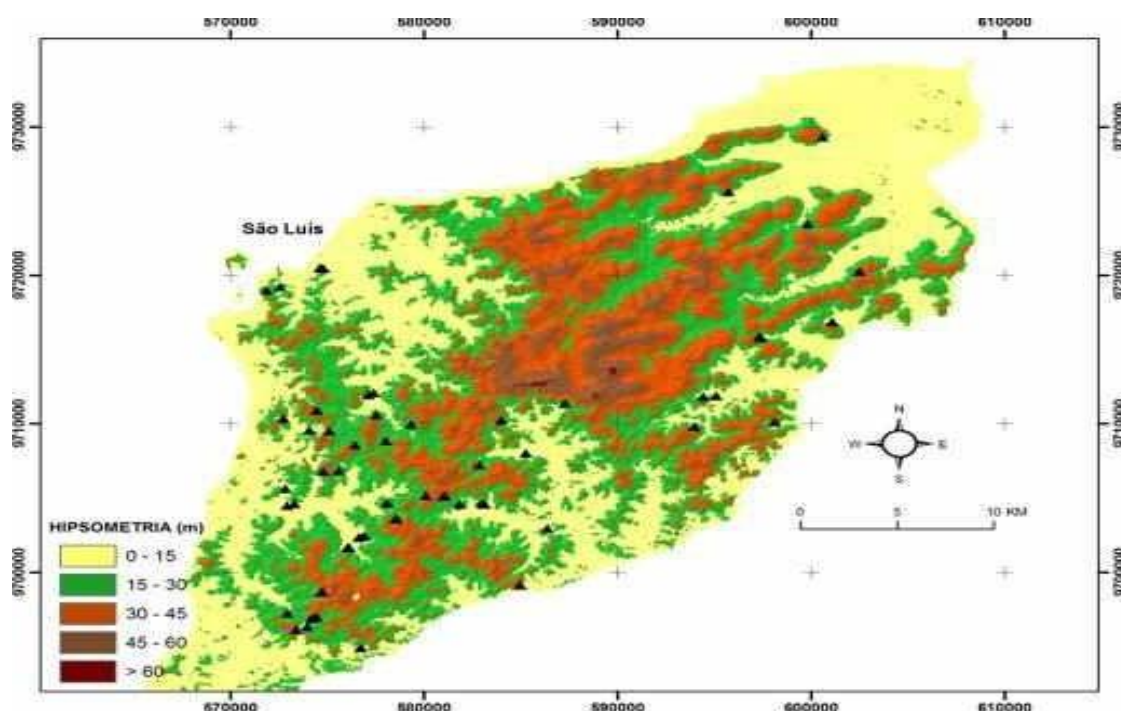
Figura 4.1 - Aspectos da geomorfologia evidenciando o domínio altimétrico (respectivas altitudes terrestres das formações geológicas) e as 47 jazidas/lavras, ou pontos/ocorrências de laterita cadastradas na ilha de São. Luís no estado do Maranhão durante os estudos de campo.
