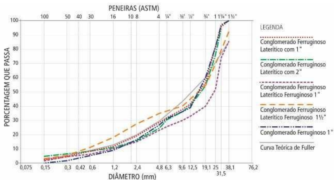
Figura 5.44 – Curvas granulométricas dos tipos petrográficos britados com abertura da mandíbula regulada com 1" - 1 1/2" - 2".
