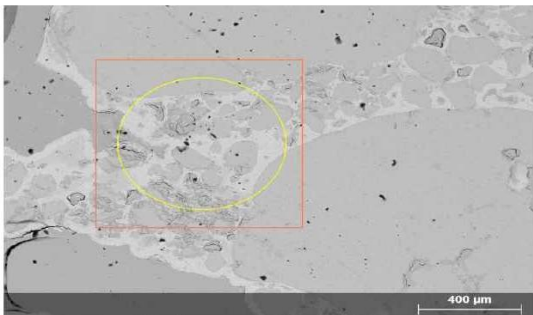
Figura 5.11 – Fotomicrografia microscópica eletrônica de varredura (MEV). Aspectos delimitados da área dentro do quadrado onde foi executado a varredura, com os resultados químicos apresentados na figura 5.12. A fotomicrografia apresenta o conjunto amostral denotando o cimento constituído de óxidos ferruginosos (hematita, goetita), sendo a fração mais esbranquiçada. A matriz é composta de quartzo, sendo representada como a fração mais escura. Na figura 400 micrômetros é equivalente a 0,4 mm.
