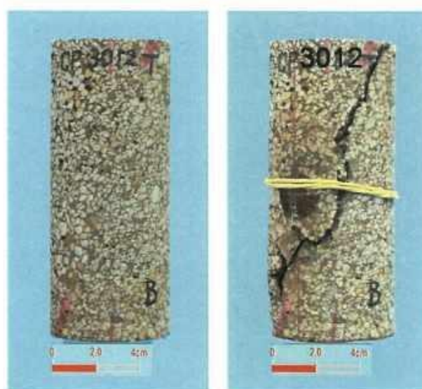
Figura 5.30 - CP 3012 antes e após o ensaio de compressão uniaxial.
