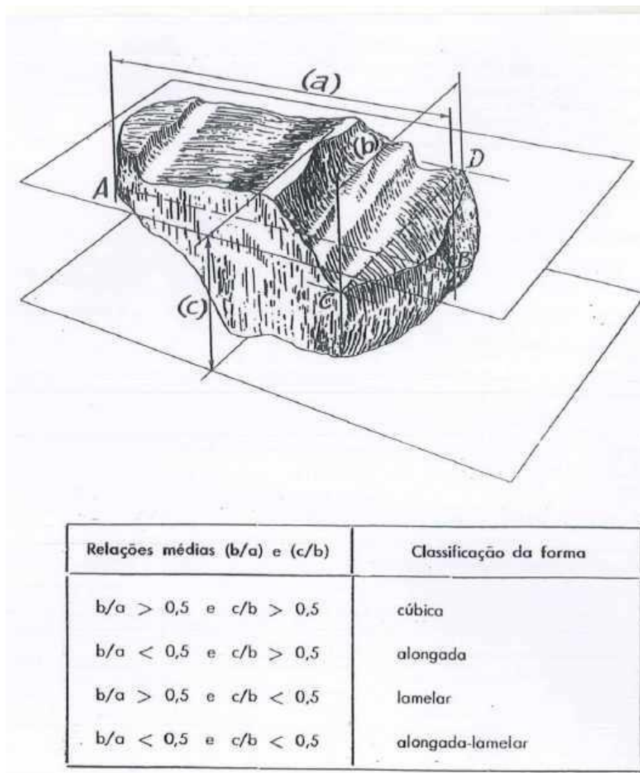
Figura 5.45 - Medidas consideradas em um fragmento de rocha para definir o índice de forma
