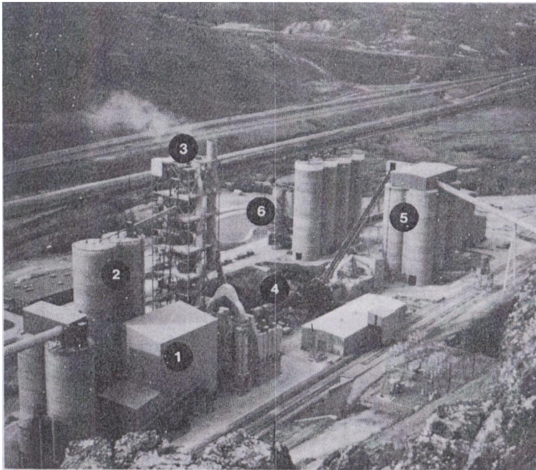
Figura 2.25 - Vista aérea da fábrica de cimento Portland Ash Grove Cement (na costa oeste dos EUA), em Durkee, Oregon: 1. moagem da matéria –prima; 2. mistura e armazenamento da farinha; 3. pré-aquecedor a suspensão; 4. forno rotativo; 5. armazenamento do clínquer; 6. moagem do cimento (Fotografia por cortesia da “Vagn Johansen, F.L. Smidth, Copenhagen, Dermark”).
