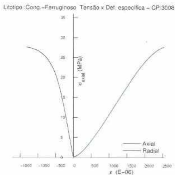
Figura 5.32 - Diagrama tensão axial versus deformação específica axial e radial do corpo de prova 3008.
