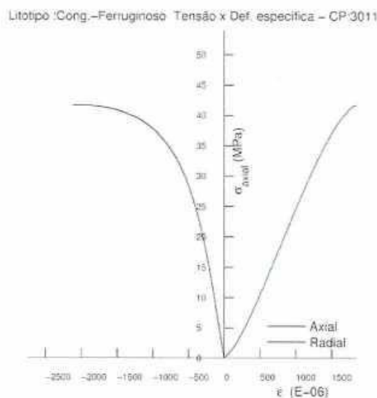
Figura 5.35 - Diagrama tensão axial versus deformação específica axial e radial do corpo de prova 3011.
