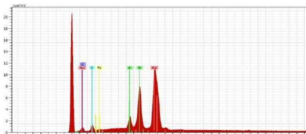
Figura 5.12 – Apresentação da energia de dispersão com detector do raio X (EDS), destacando-se os constituintes minerais da amostra da Figura 5.11.
