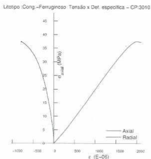
Figura 5.34 - Diagrama tensão axial versus deformação específica axial e radial do corpo de prova 3010.
