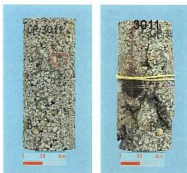
Figura 5.29 - CP 3011 antes e após o ensaio de compressão uniaxial.
