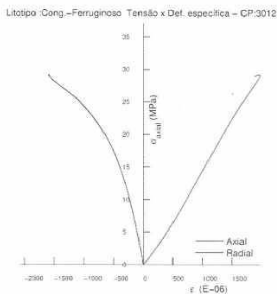
Figura 5.36 - Diagrama tensão axial versus deformação específica axial e radial do corpo de prova 3012.
