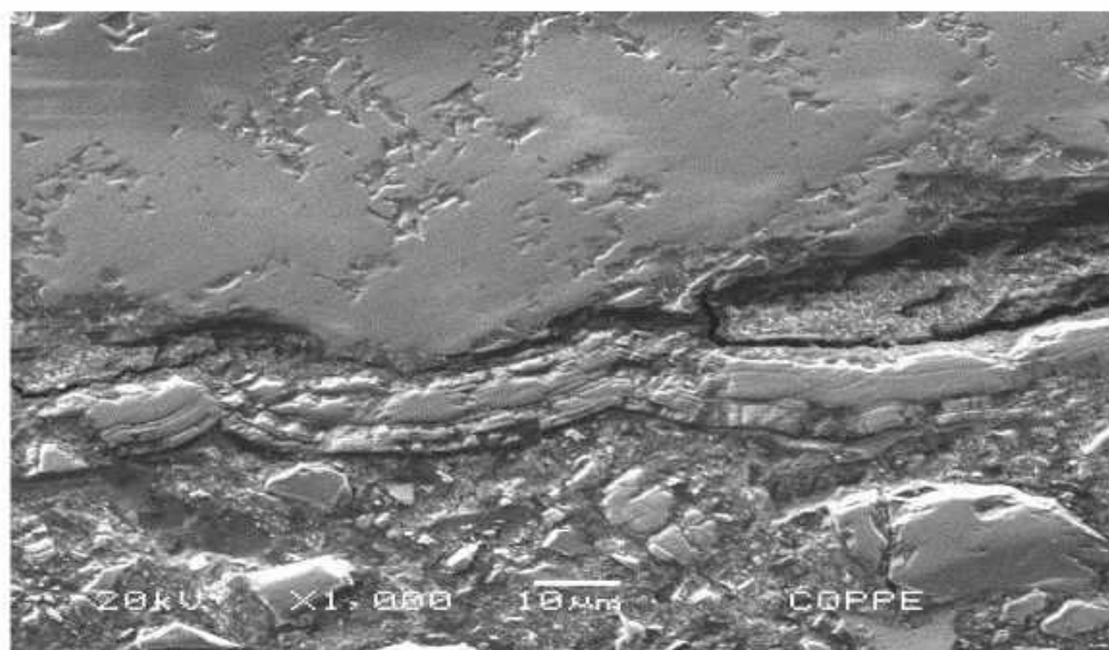
Figura 5.15 – Detalhe da foto Figura 5.14 mostrando o contraste divisório entre o quartzo e o cimento ferruginoso.
