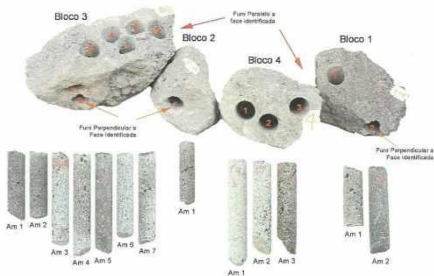
Figura 5.23 - Blocos de rocha 1 a 4 e as 13 (treze) amostras retiradas no Laboratório de Mecânica das Rochas. Litotipo: conglomerado ferruginoso (laterita).
