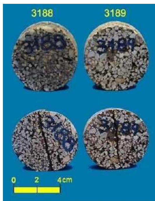
Figura 5.43 - Vista dos corpos de prova cp3188 e cp3189 antes e após ensaio de compressão puntiforme na direção axial. Bloco 02 AM 01 e litotipo conglomerado ferruginoso.
