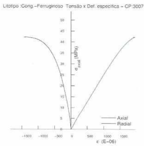
Figura 5.31 - Diagrama tensão axial versus deformação específica axial e radial do corpo de prova 3007.
