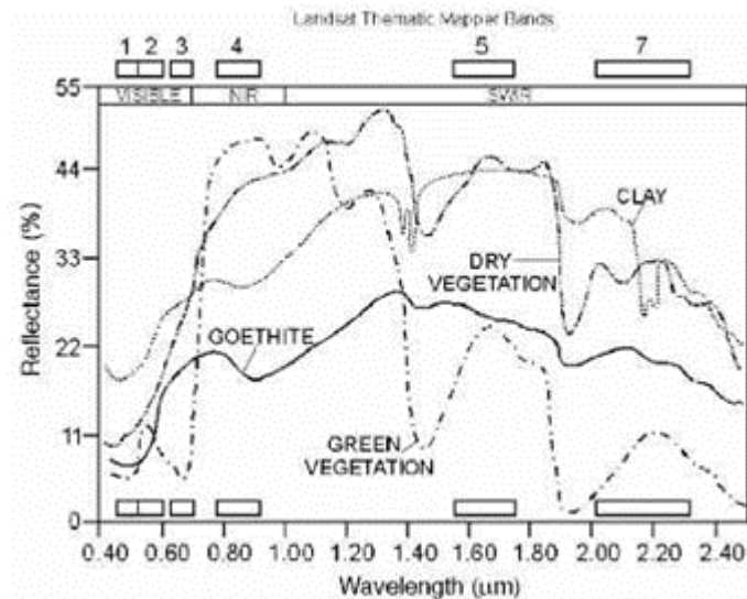
Figura 5.2 - Assinaturas espectrais de óxido de ferro (goethita), vegetação e argila. Extraído de Carranza & Hale (2002). Notar que a goethita (ou a hematita) mostra baixa resposta nos canais TM 1, 2 e 4 e alta resposta nos canais TM 3, 5 e 7 do LANDSAT5-TM.
