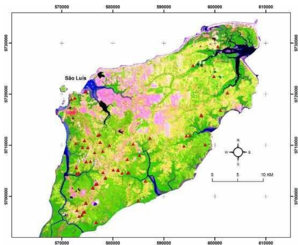
Figura 5.3 - Composição colorida 7R4G3B realçada, com indicação dos pontos/jazidas/lavras onde ocorrem as lateritas ferruginosas (triângulos vermelhos).
