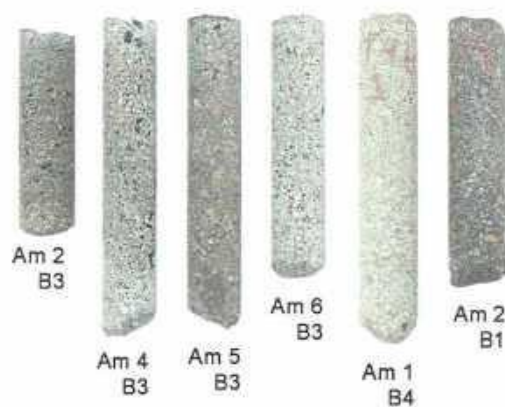
Figura 5.24 - Amostras adequadas para os ensaios de compressão. Litotipo: conglomerado ferruginoso (laterita).
