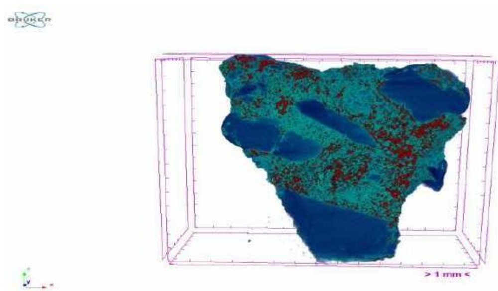
Figura 5.18 - Microtomografia computadorizada com raio X, análise da porosidade, espessura e distribuição com vista 3D.
