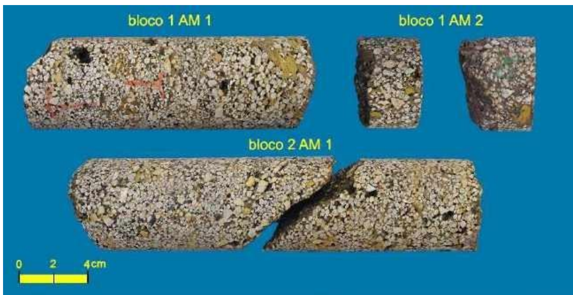
Figura 5.37 - Amostras extraídas de blocos de rocha no laboratório de mecânica das rochas (LMR), no ano de 2016, correspondentes aos blocos 1 e 2, sendo AM1 e AM2 do bloco 1e AM1 do bloco 2.
