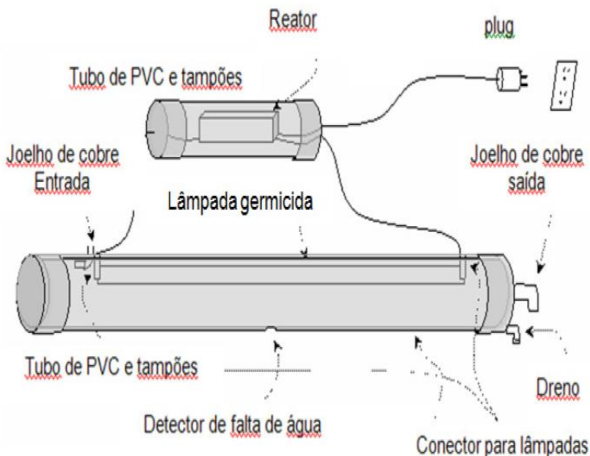
Figura 06 – Imagem de proposta do protótipo do Tubo UV a ser confeccionado com materiais da região estudada nesta pesquisa analisando sua aceitabilidade, viabilidade econômica e operacional mediante adaptação as condições locais.
