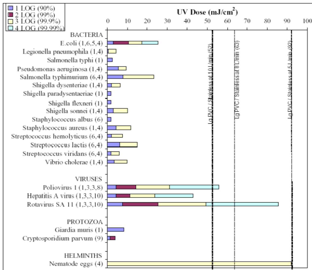
Quadro 04 – Comparativo de eficiência da aplicação de doses de radiação UV( \text{mJ}/\text{cm}^2 ) destinadas a eliminação de patógenos conforme vazões de 10, 08 e 05 litros de água/minuto (L/min) tratadas no Tubo UV.
