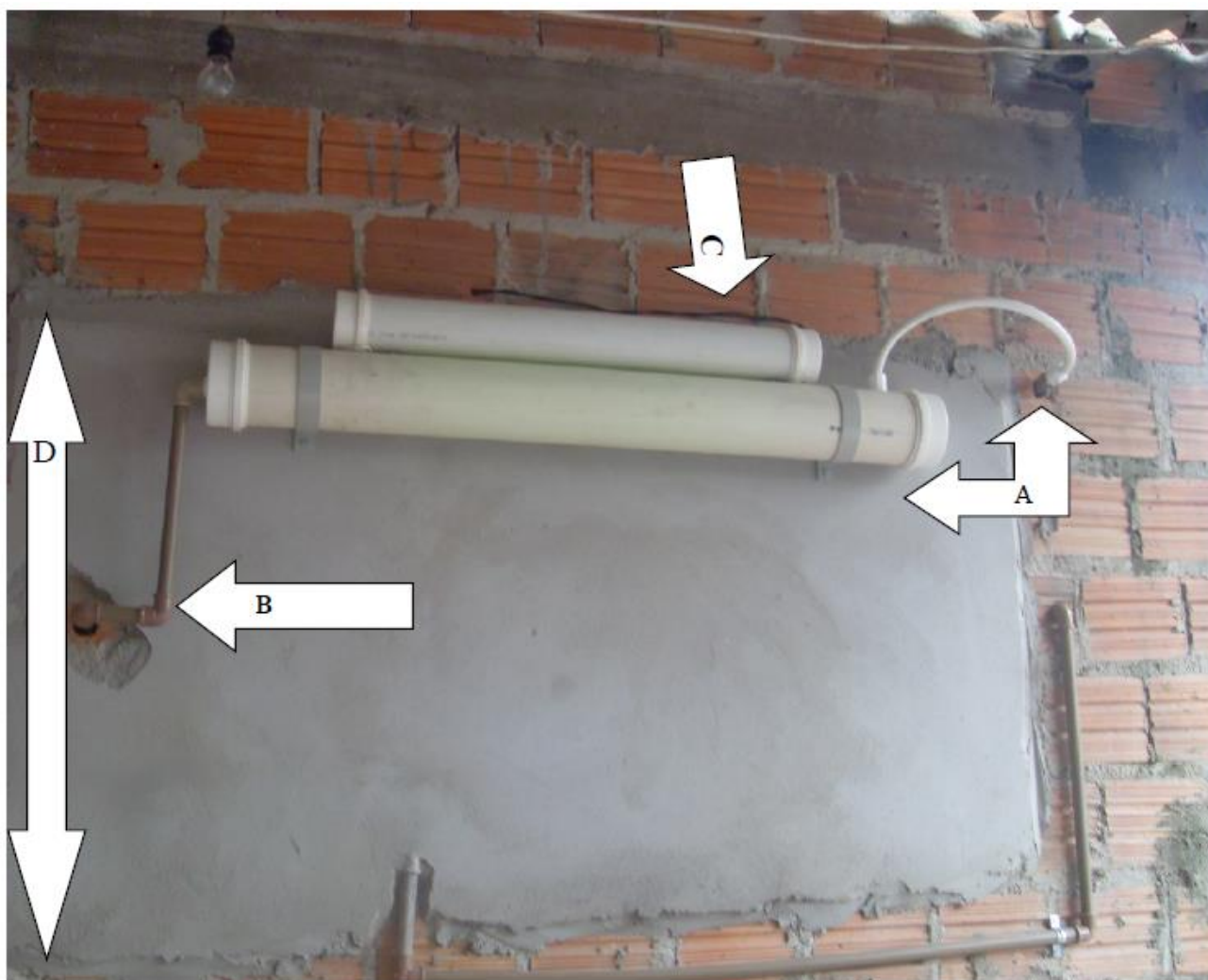
Figura 42 – Imagens do Tubo UV instalado na residência do Sr. Francisco e fixado na parte externa revestida da residência (D), mostrando a entrada de água não tratada para o equipamento (A), entrada da água já tratada para o interior da residência (B) e parte da fiação elétrica que alimenta a lâmpada UV (C) com controle do acionamento no interior da casa por solicitação do próprio morador que, inicialmente, julgou não muito atraente o design do protótipo. Casa localizada no assentamento rural Boa Esperança – Zé Doca, Maranhão, Brasil.
