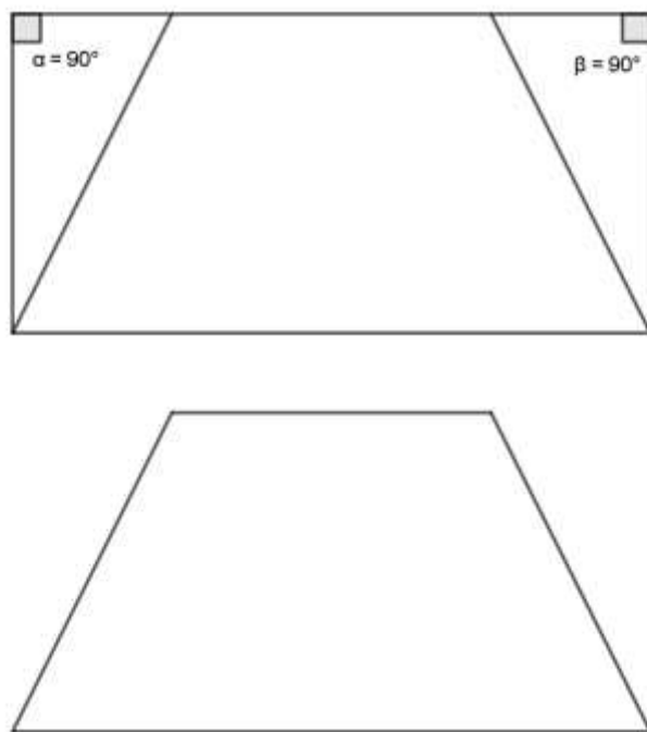
Figura 28 - Trapézio.
