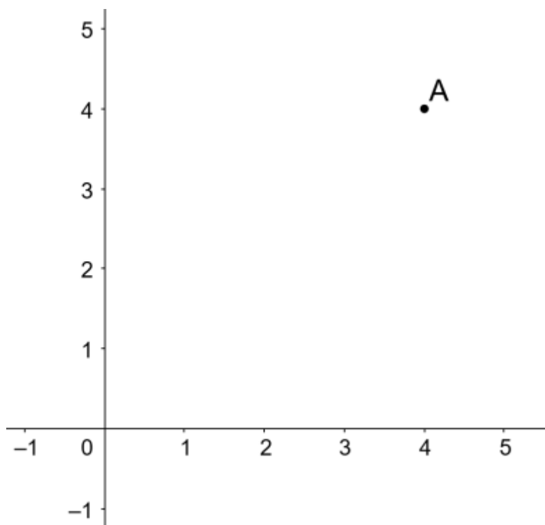
Figura 11 - Ponto.
