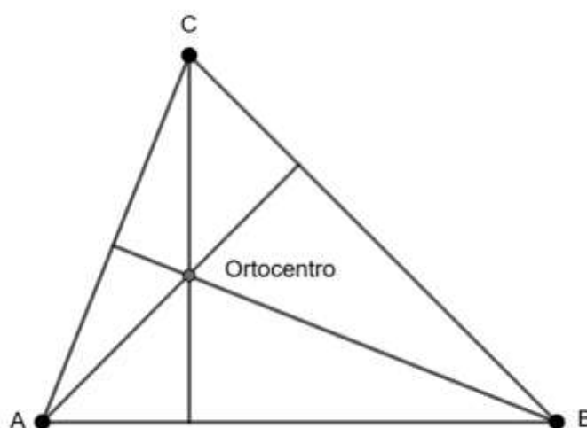
Figura 63 - Ortocentro.
