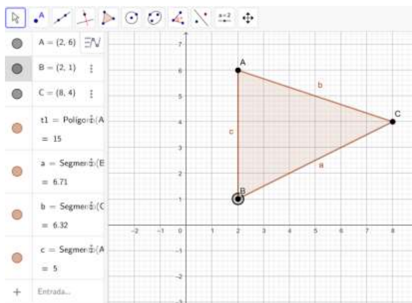
Figura 36 - GeoGebra.
