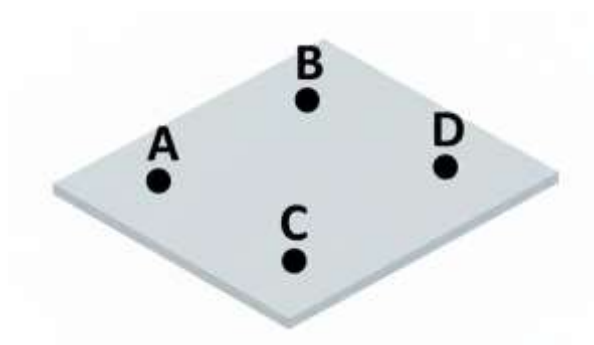
Figura 19 - Pontos Coplanares
