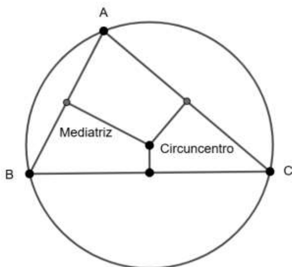
Figura 61 - Circuncentro.
