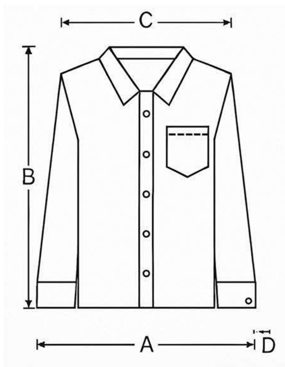
Figura 9 - Moda.
