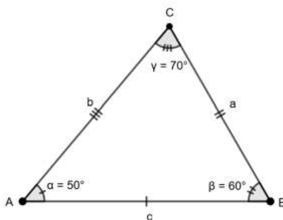
Figura 44 - Triângulo Acutângulo.
