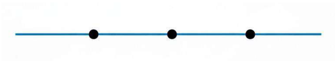
Figura 18 - Pontos Colineares.
