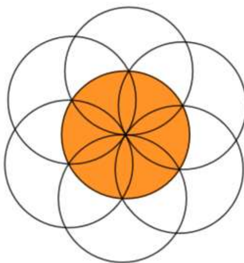
Figura 70 - Mandala Circular.
