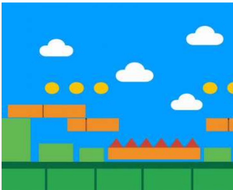
Figura 7 - Gráfico 2D.
