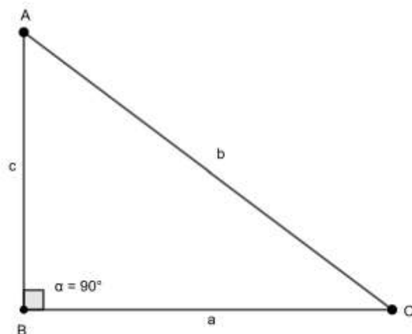
Figura 45 - Triângulo Retângulo.
