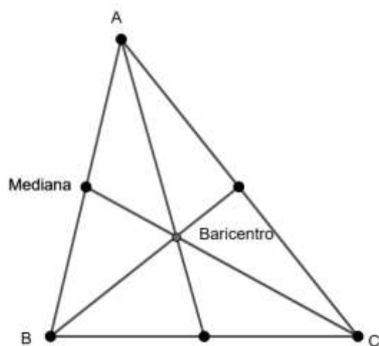
Figura 62 - Baricentro.
