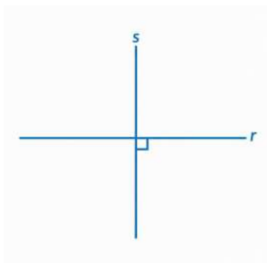
Figura 21 - Retas Perpendiculares.
