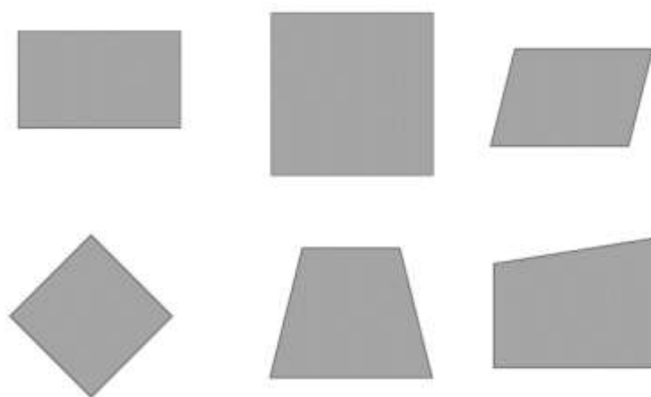
Figura 67 – Quadriláteros
