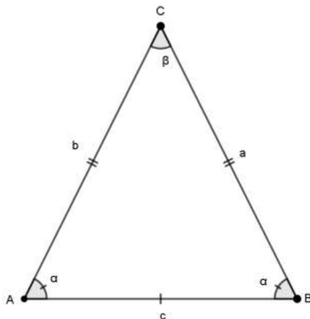
Figura 42 - Triângulo Isósceles.
